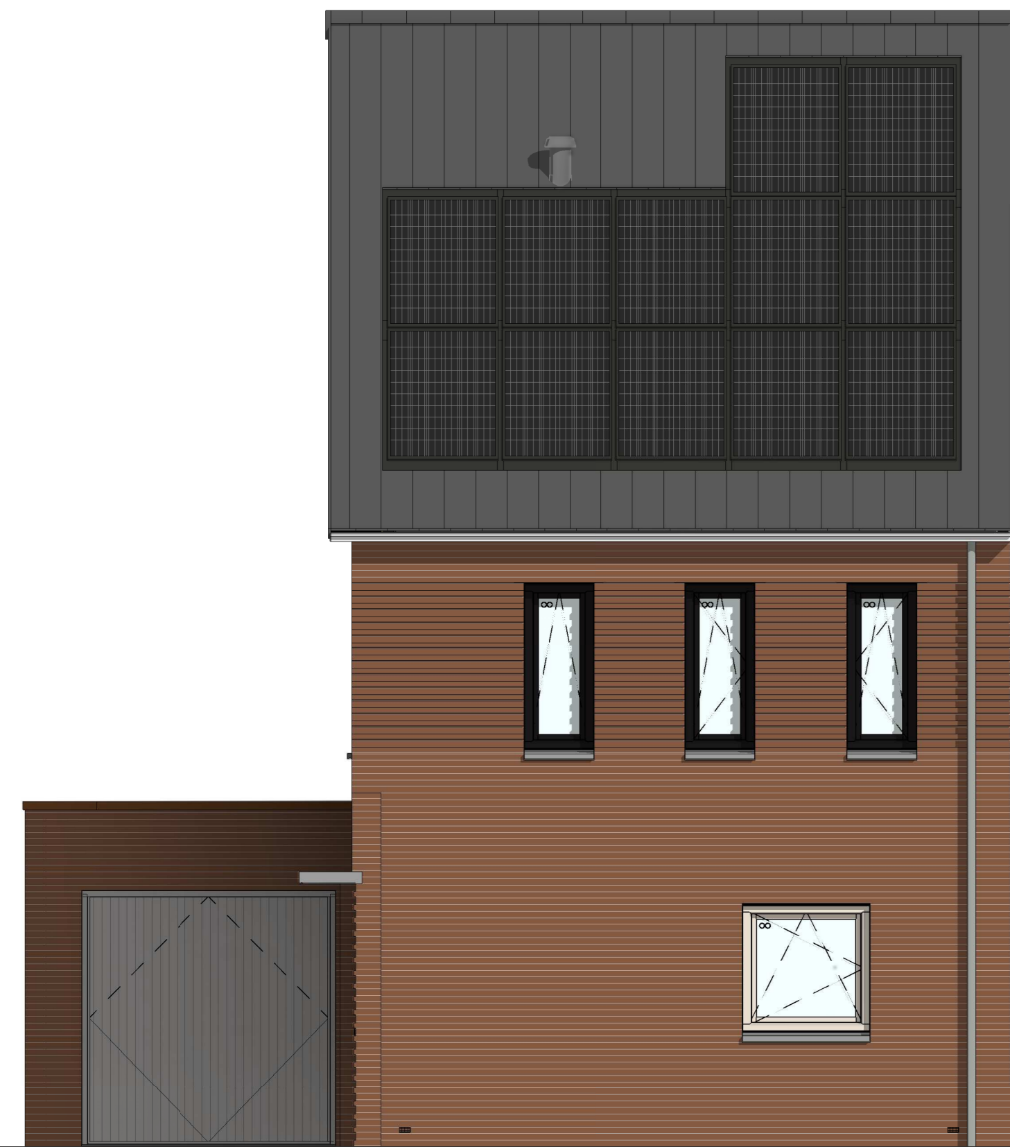
VG5001 - Voorgevel in basis uitvoering
