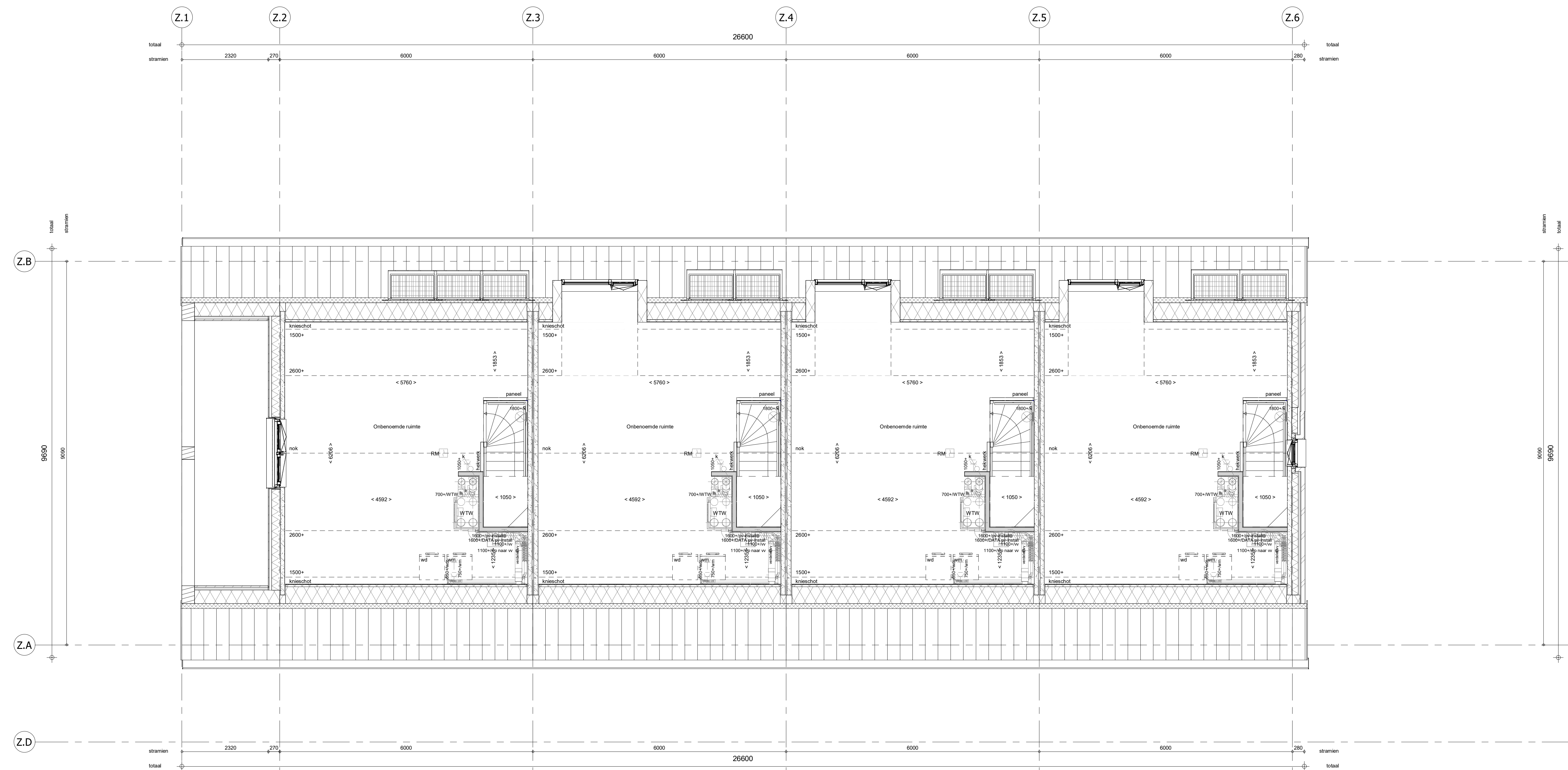
2e verdieping 1 : 50
