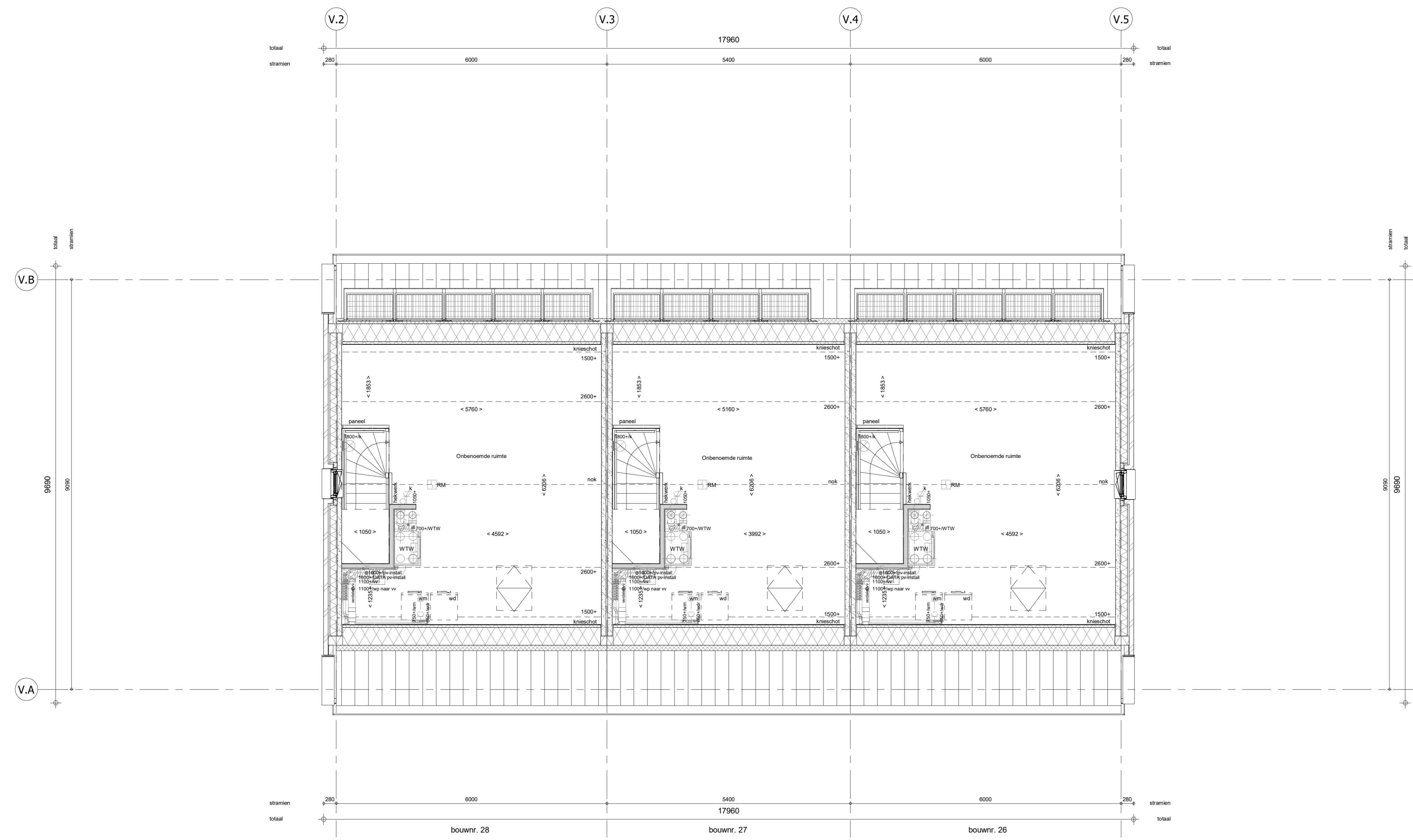
2e verdieping 1 : 50
