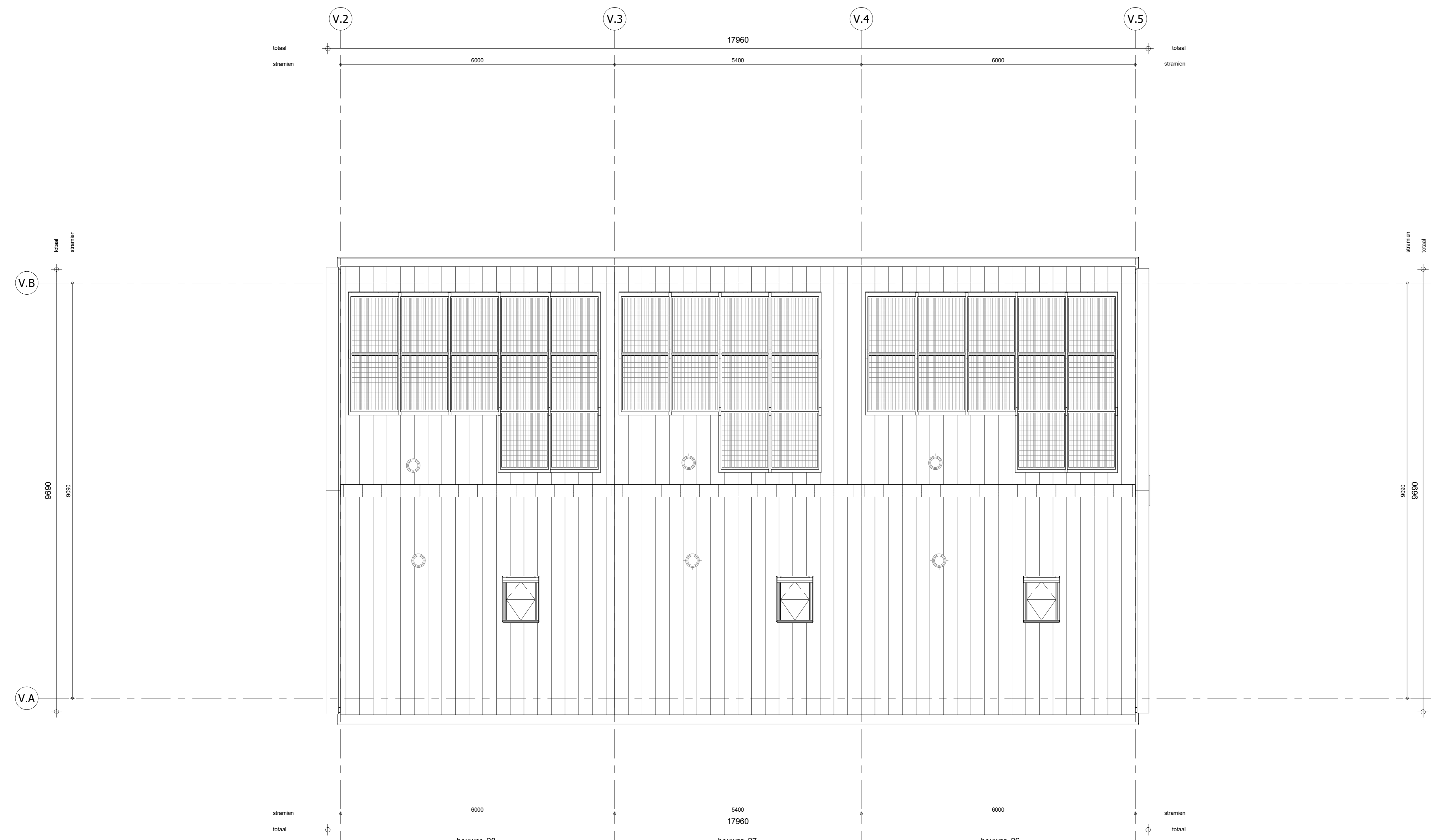
Dakaanzicht 1 : 50
