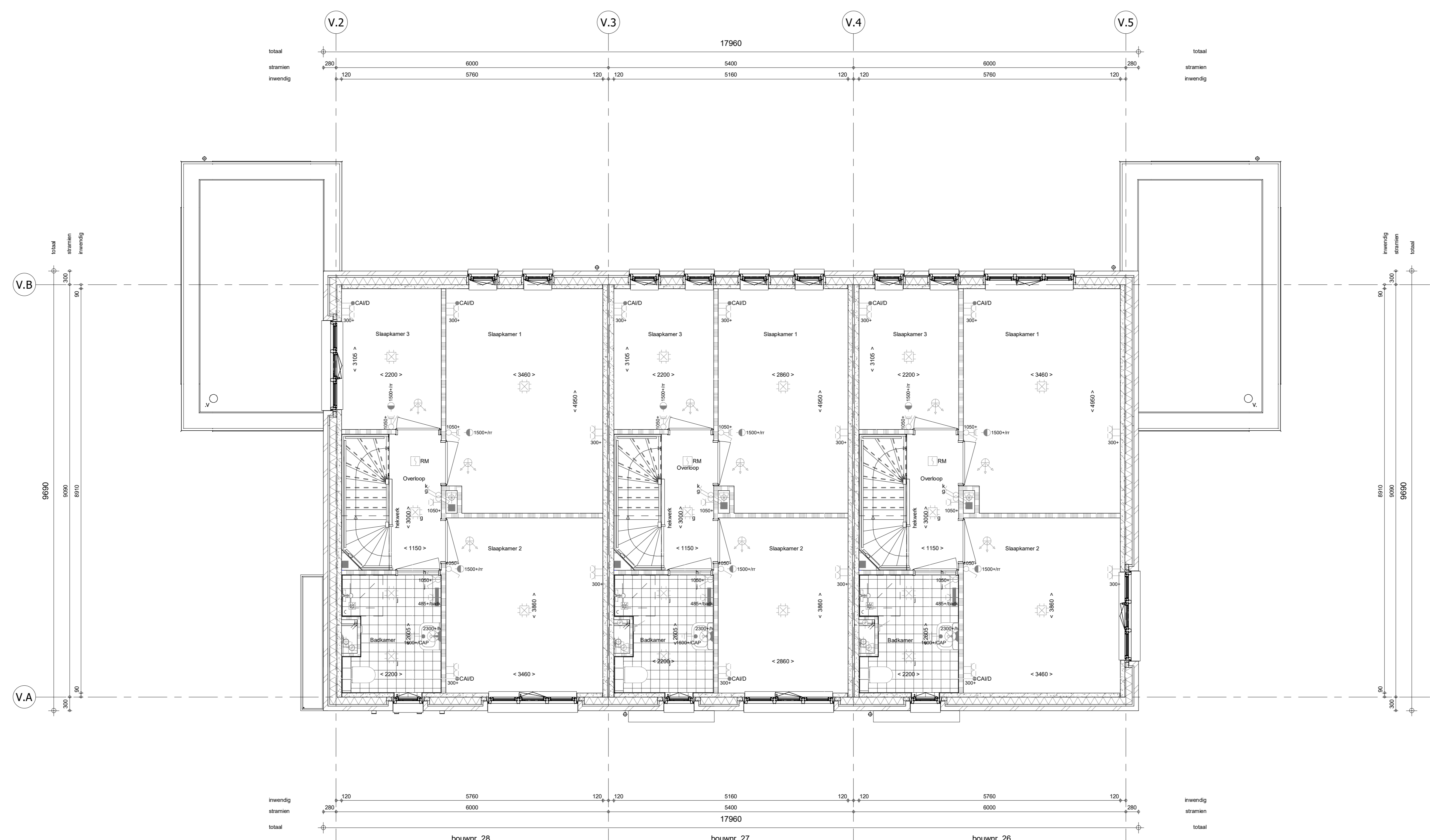
1e verdieping 1 : 50
