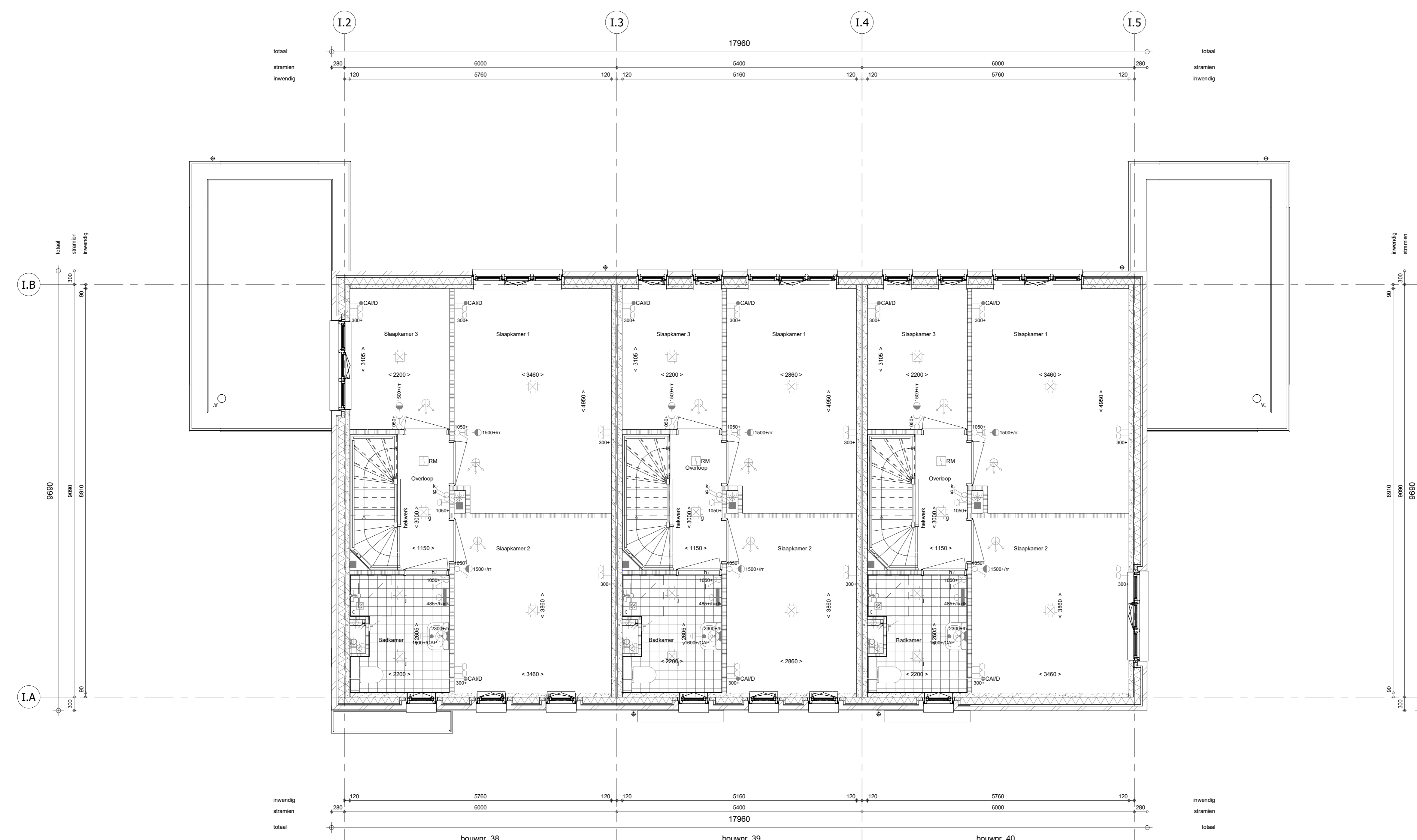
1e verdieping 1 : 50
