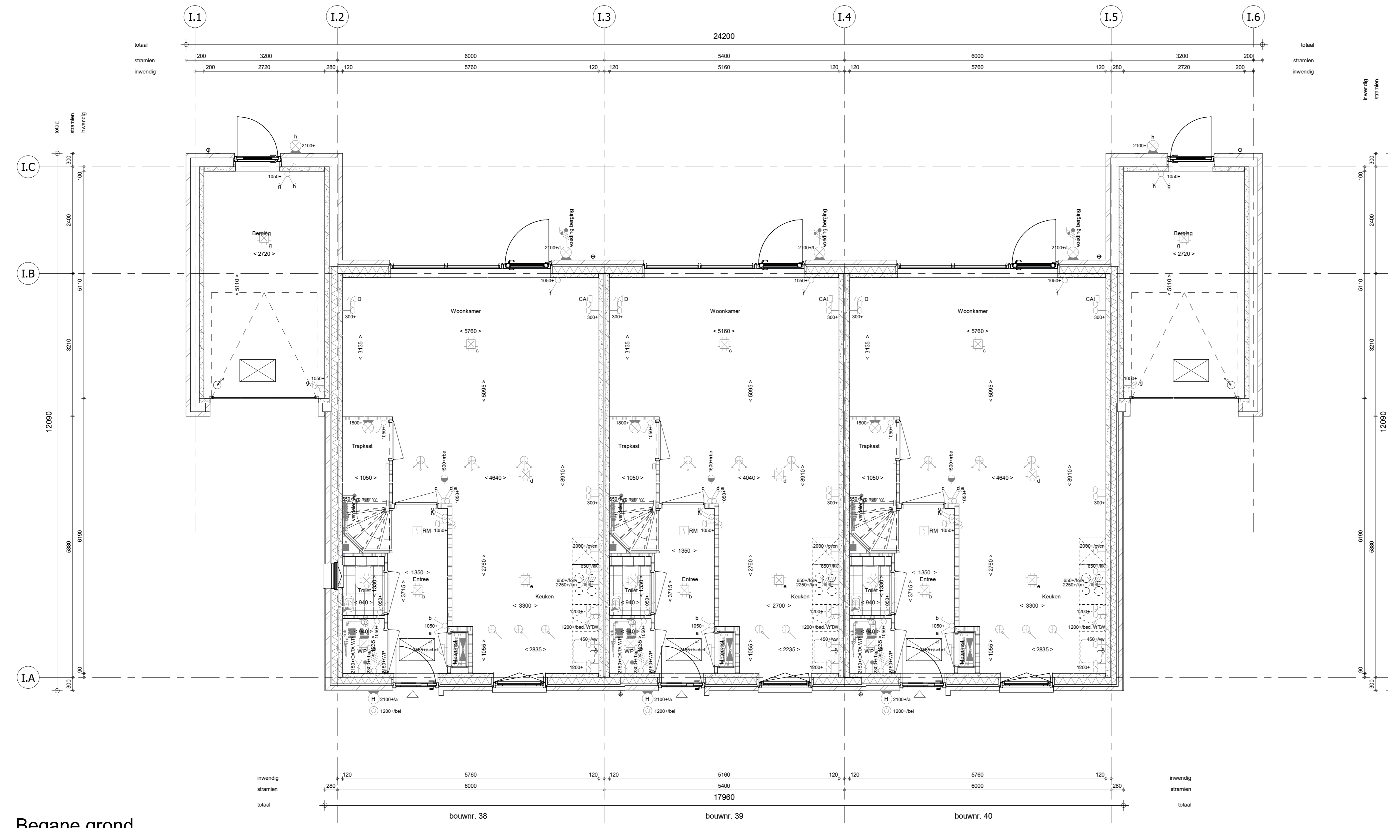
Begane grond 1 : 50
