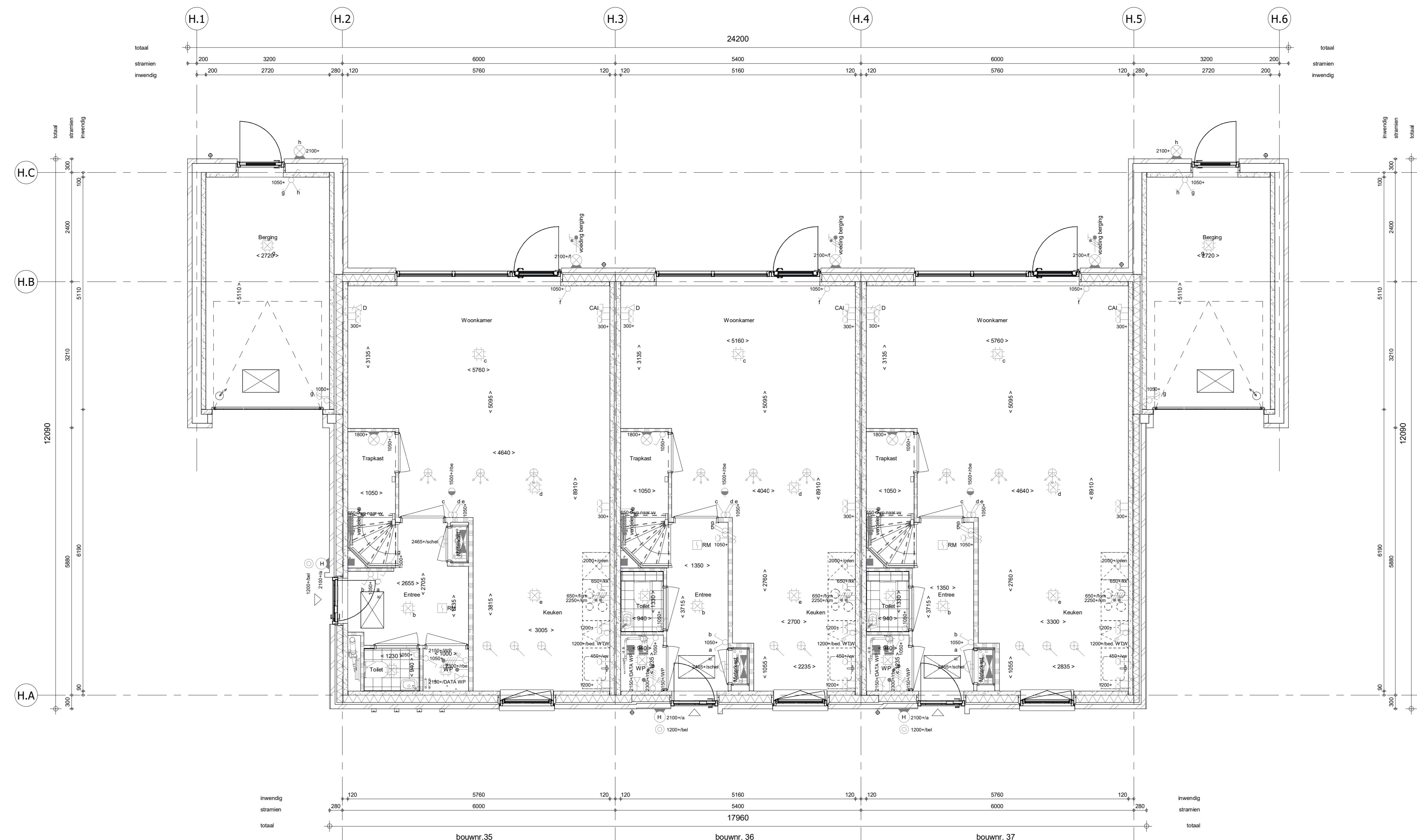
Begane grond 1 : 50
