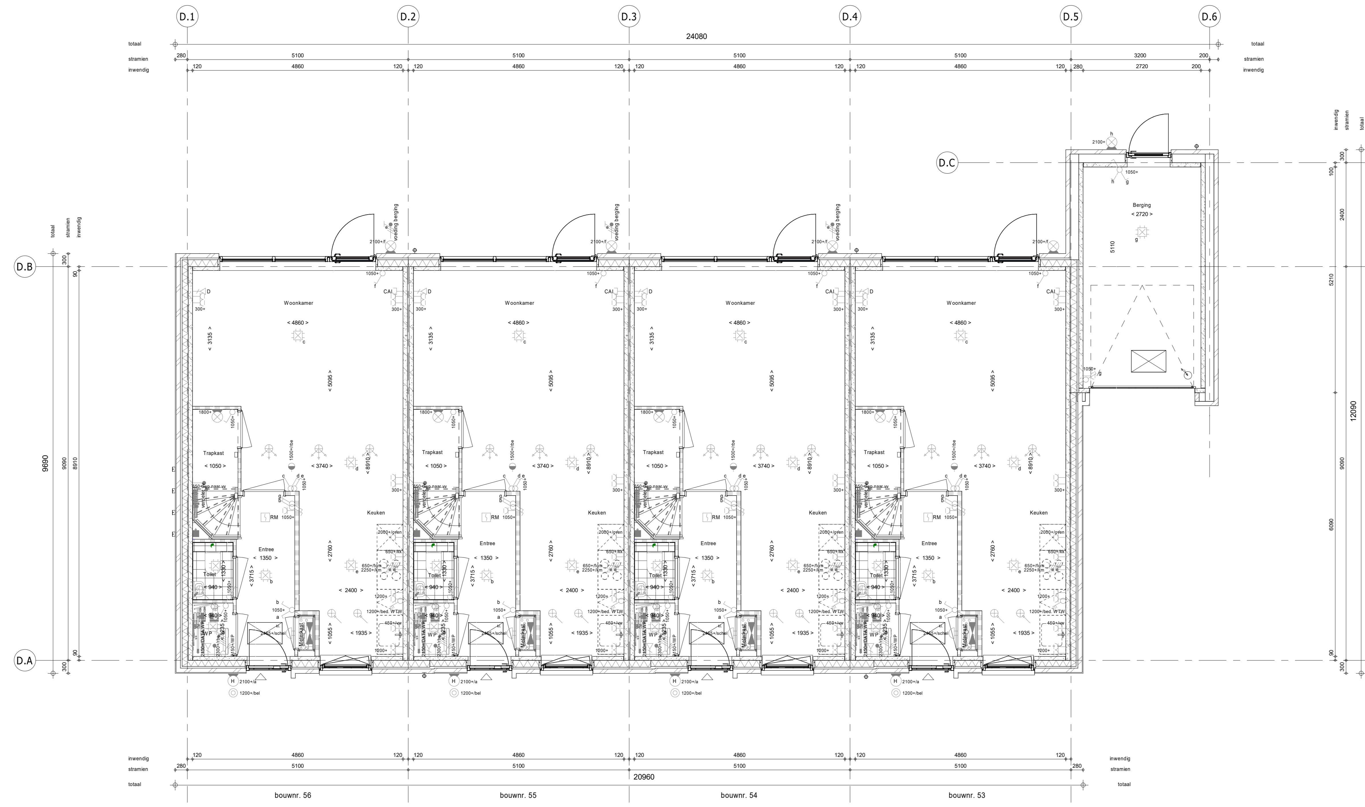
Begane grond 1 : 50
