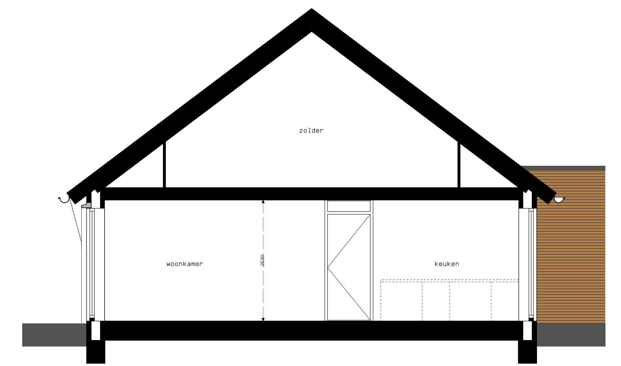
Bnr 24 DOORSNEDE 1:50
