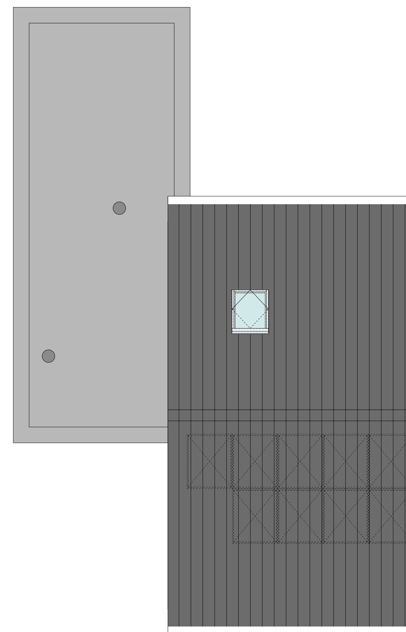
B. 11-6000 Bnr 24 DAKAANZICHT 1:50
