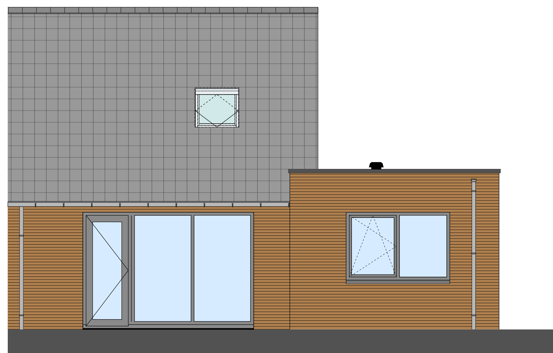
B. 11-6000 Bnr 24 ACHTERGEVEL 1:50
