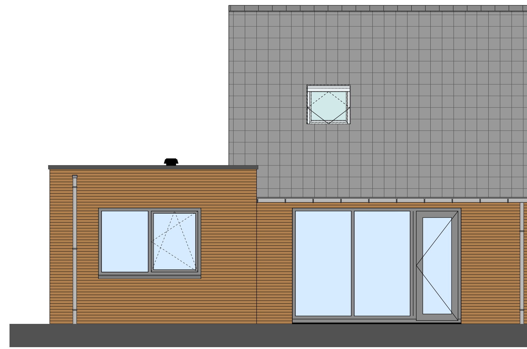
B. 11-6000 BNR 23 ACHTERGEVEL 1:50
