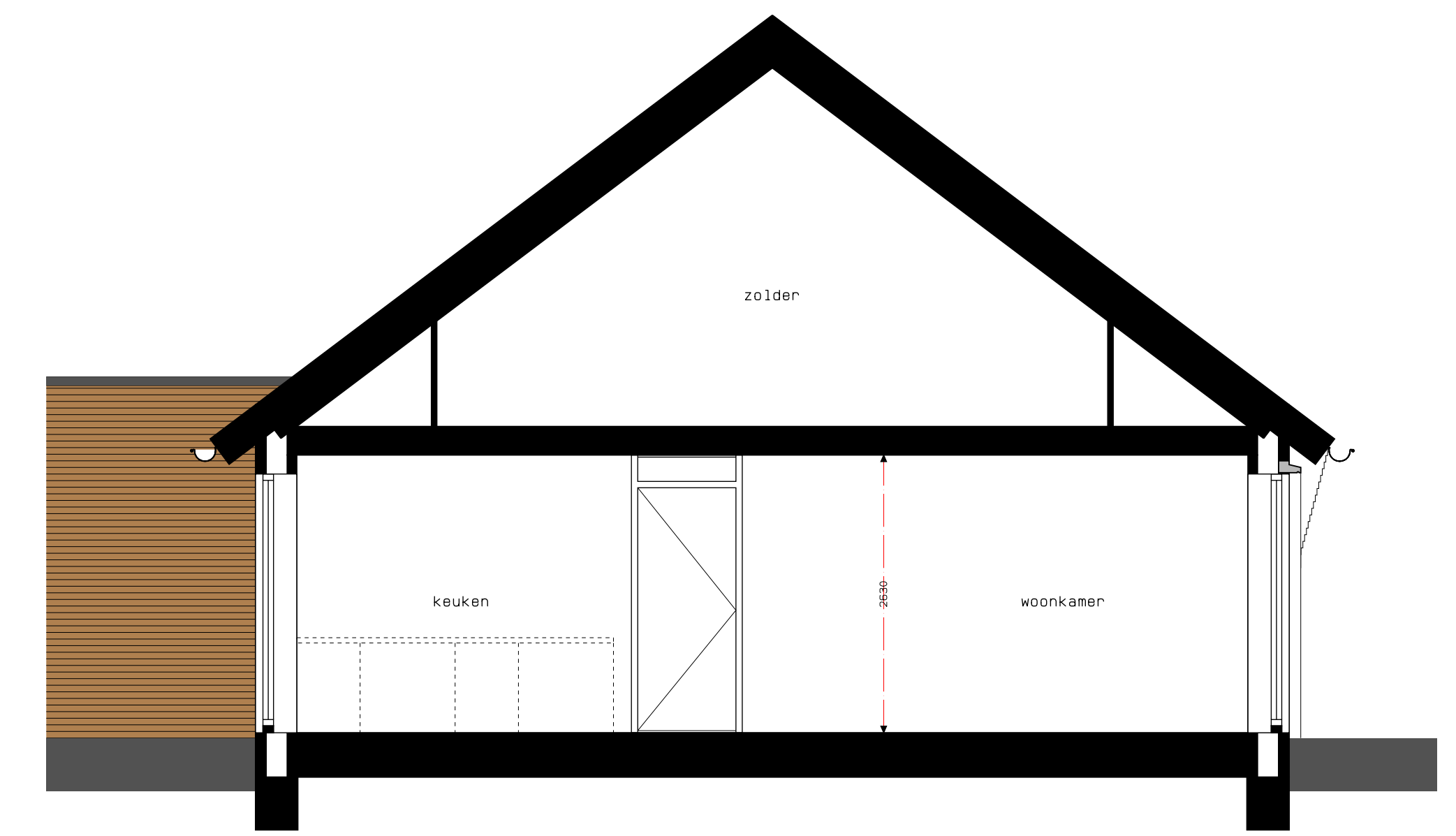
BNR 23 DOORSNEDE 1:50
